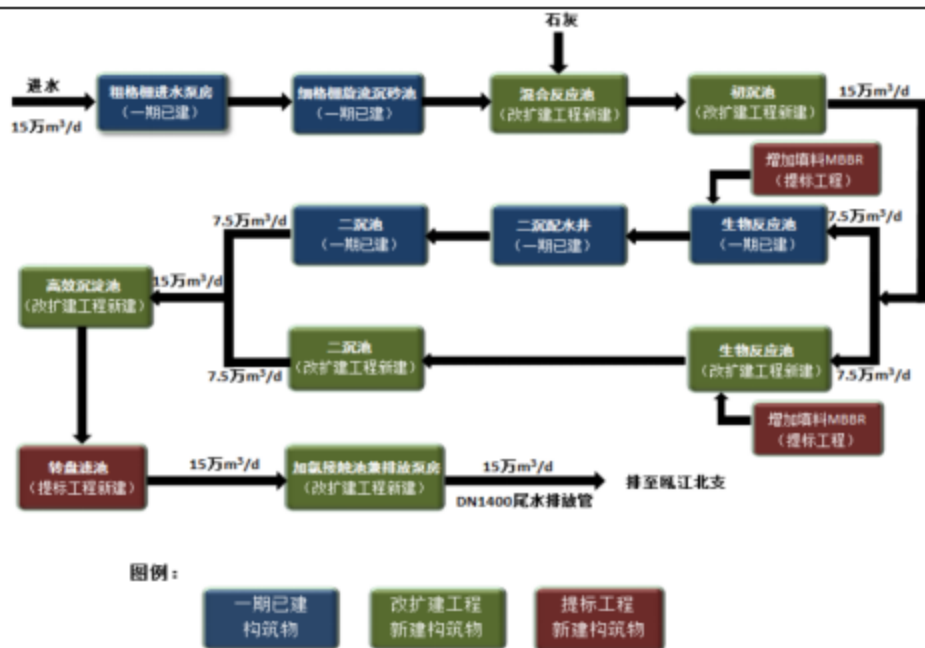
图 4-1 水处理工艺流程示意图
